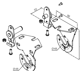
525.10072 max 40 Nm
