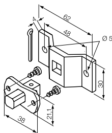
523.10012
