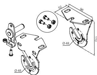
525.10071 max 30 Nm
