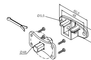
525.10061 max 30 Nm
